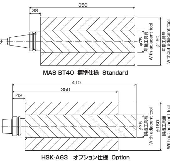
ATC最大工具寸法図 ATC maximum tool dimension
